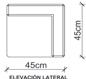
ELEVACIÓN LATERAL
